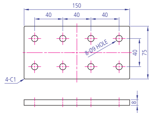
YKBK-DC OS 75x150 Code : YKBK-DOS75150 Code : YKBK-DOS75150B(흑착)
