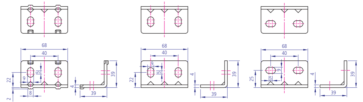
YKBK-S LG801 Code : YKBK-SLG801
