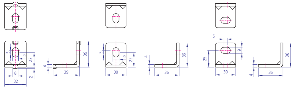
YKBK-S LG401 Code : YKBK-SLG401
