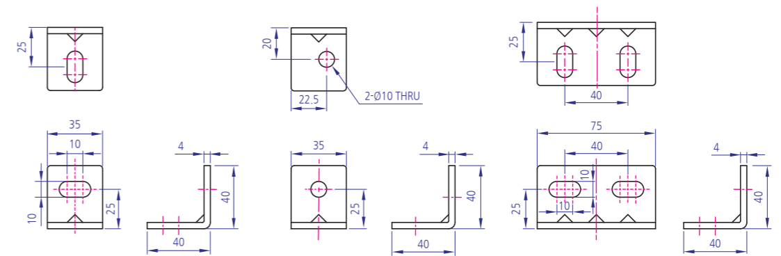
YKBK-S LD40*35(SLOT10) Code : YKBK-SLD4035
