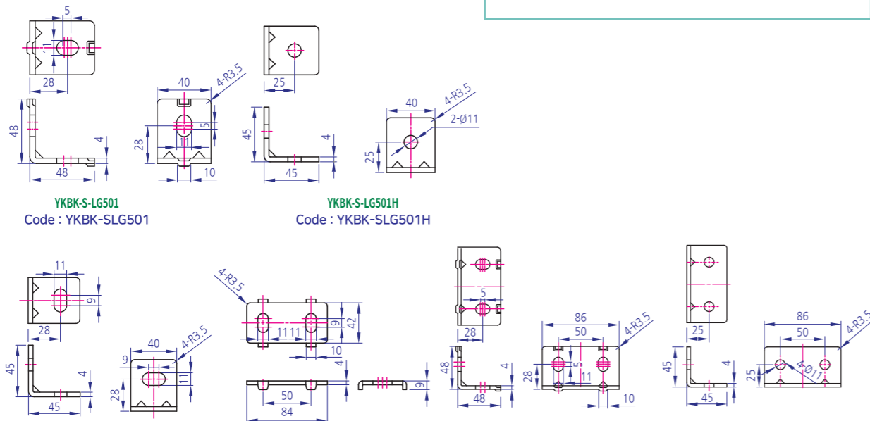
YKBK-S LG503 Code : YKBK-SLG503
