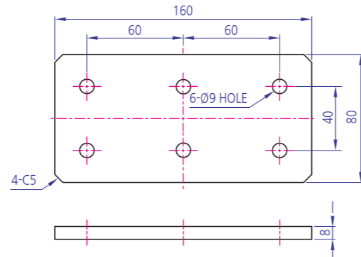
YKBK-DC OS 80x160 Code : YKBK-DOS80160
