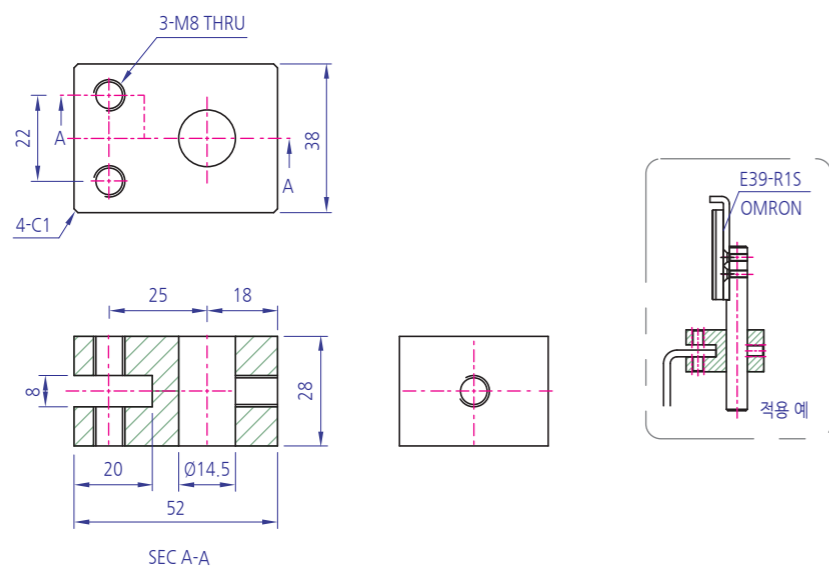
SEC A-A
