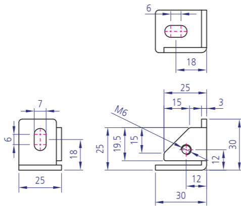
YKBK-S T30*25(M6) Code : YKBK-ST3025A
