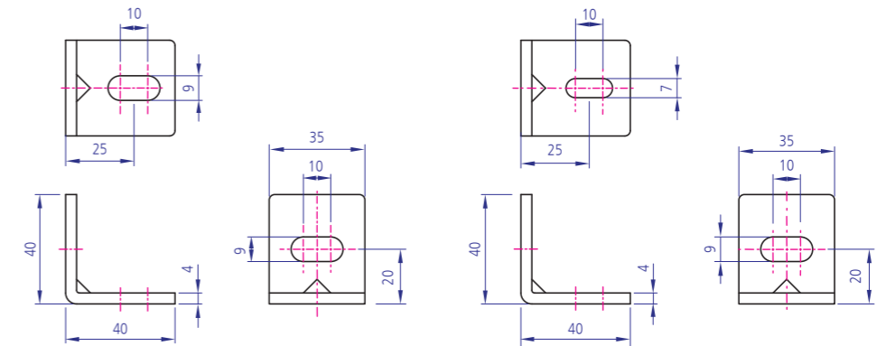
YKBK-S 태양광 40*35 (SL9*10)
