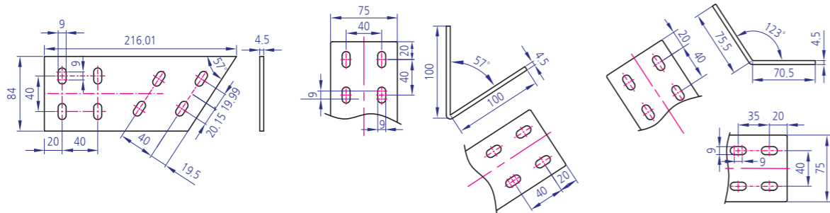
YKBK-S 84*216*4.5T Code : YKBK-SS84216
