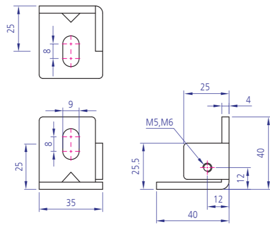
YKBK-S T40*35(M5,M6) Code : YKBK-ST4035
